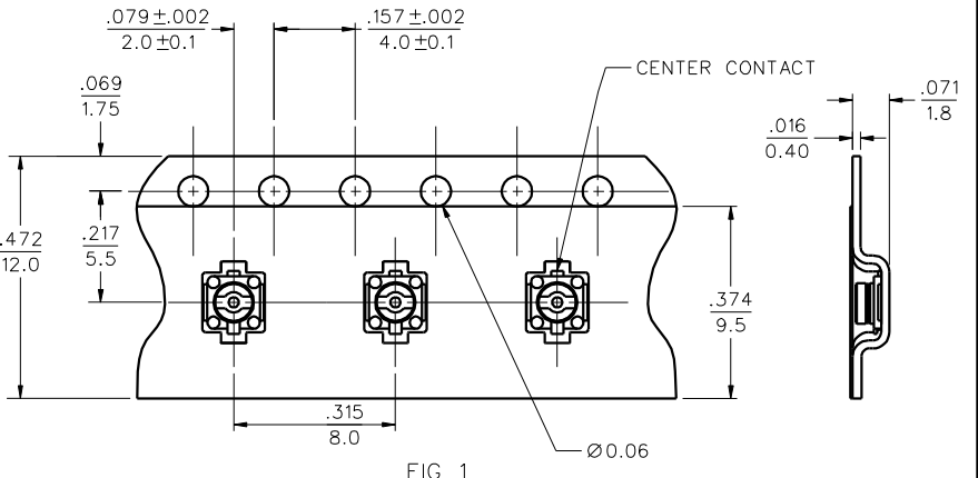
FIG 1 5:1
