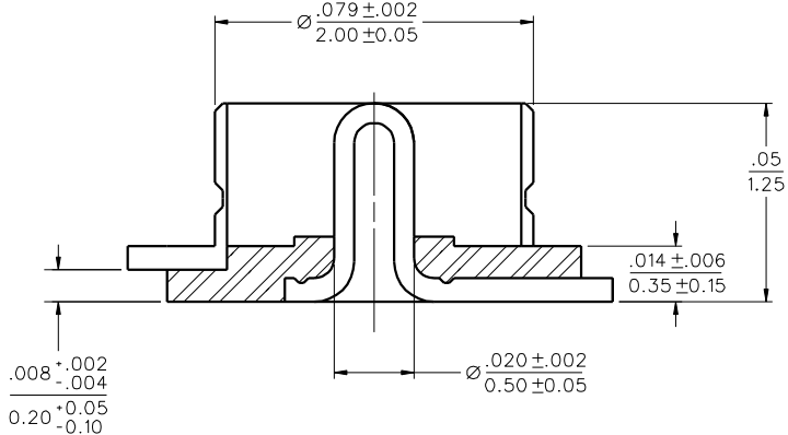
SECTION A-A 40:1
