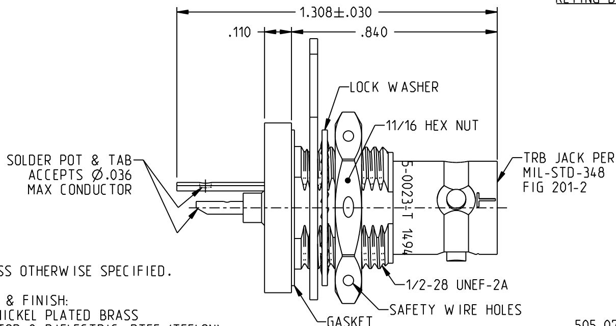
505-0745-1 SHOWN
