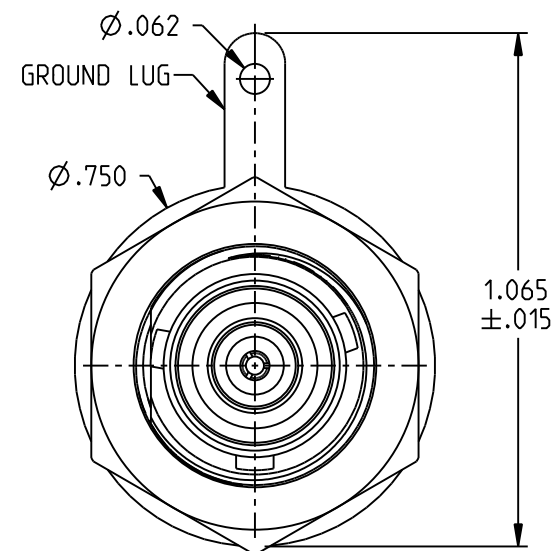
505-0745-1 SHOWN
